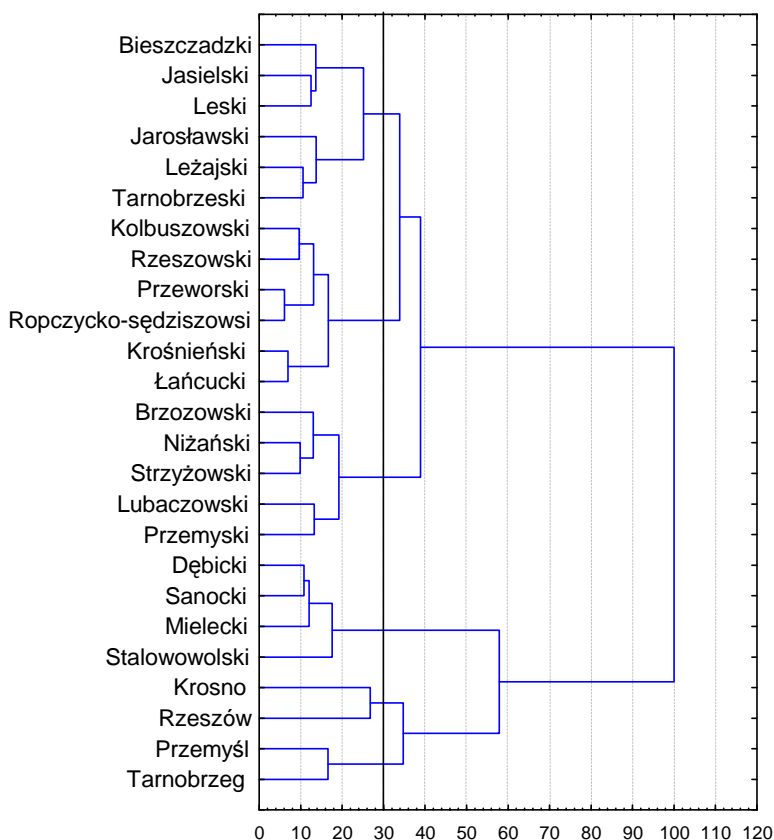
Wykres 31. Grupowanie powiatów metodą Warda w zakresie rynku pracy w 2009 r.
